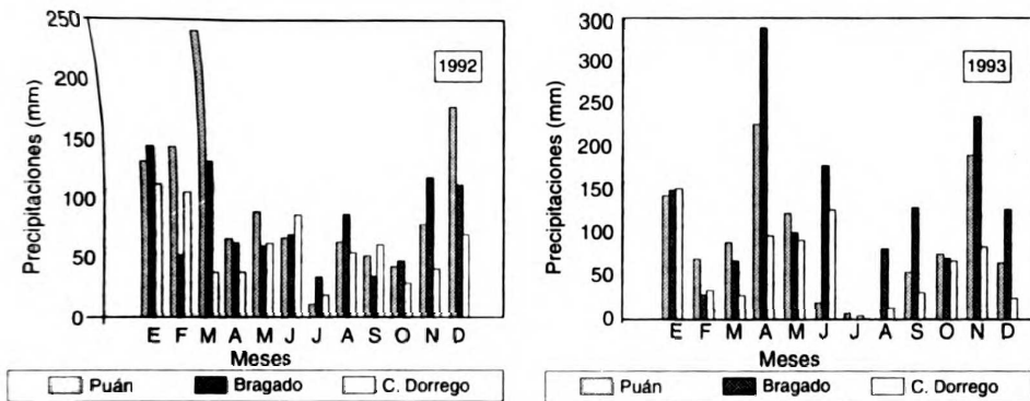
Figura 2. Precipitaciones en las localidades de Puán, Bragado y C. Dorrego en 1992 (a) y 1993 (b). Rainfall in Puán, Bragado and C. Dorrego in 1992 (a) and 1993 (b).
