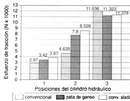
Figura 2. Esfuerzos de tracción registrados para las diferentes posiciones del cilindro hidráulico de control remoto.
