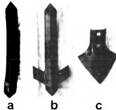
Foto 1. Rejas utilizadas en los ensayos: a) Convencional, b) Convencional alada, c) Pata de ganso
