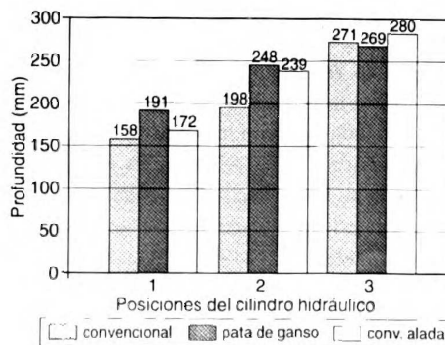
Figura 1. Profundidades de trabajo alcanzadas por las diferentes rejas.
