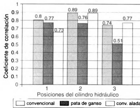
Figura 4. Correlación entre áreas medidas y calculadas.
