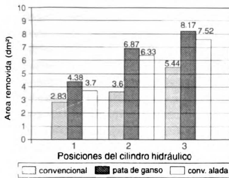
Figura 3. Áreas removidas para los distintos tratamientos.
