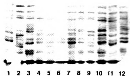
Figura 2: Patrones de gluteninas de alto peso molecular obtenidos por electroforesis. De izquierda a derecha: 1:Pampa INTA, 2:Buck Chamamé, 3:Klein Criollo, 4:SWM nº 1285, 5:Buck Patacón, 6:Cooperación Nanihue, 7:Granero INTA, 8:Buck Napucá, 9:Buck Pucarà, 10:Bonaerense Pasuco, 11:Pampa INTA, 12:SWM nº 6629.
