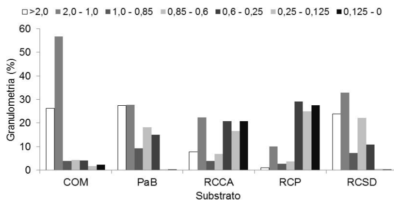
Figura 1. Distribuição do tamanho de partículas (%) de materiais utilizados como substrato. COM: substrato comercial; PaB: paú de buri; RCCA: resíduo da carnaúba com casca de arroz; RCP: resíduo da carnaúba em pó; RCSD: resíduo da carnaúba semidecomposta.
