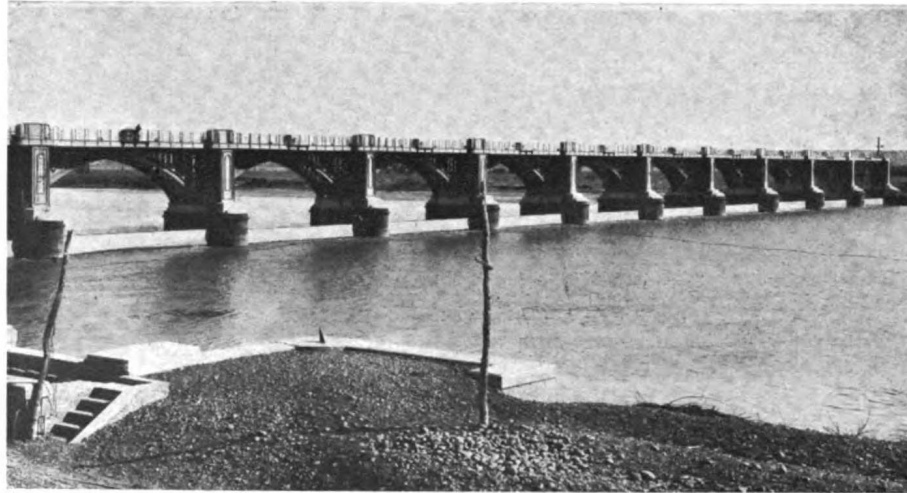
Dique.—Puente sobre el Río Neuquen desde donde arranca el canal de riego para el valle superior del Río Negro. La superficie regable es de 55,000 hectareas la que se halla recorrida por una abundante red de canales primarios, secundarios y terciarios que llevan el agua a las distintas propiedades.
