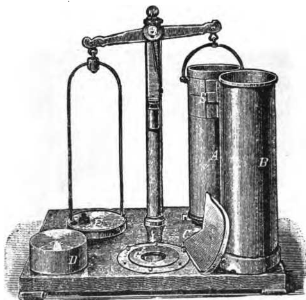
Fig. 1. Aparato para la determinación del peso del hectólitro.
