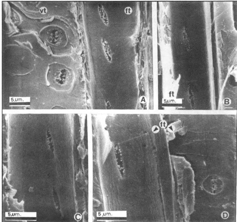
Figura 3. A-D, E. dunnii Maiden: puntuaciones ornadas en fibrotraqueidas, micrografías con MEB: A, puntuaciones ornadas en traqueidas vasicéntricas y fibrotraqueidas: vista externa e interna, respectivamente; B-D, puntuaciones ornadas en fibrotraqueidas: B-C, vista interna, D, vista interna y externa, detalle ft: fibrotraqueidas; vt: traqueidas vasicéntricas.
