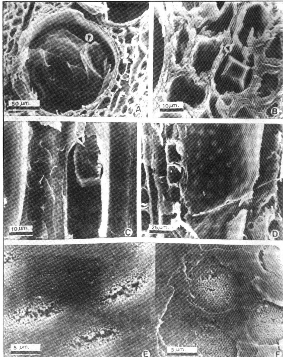
Figura 1. A-F, E. dunnii Maiden: micrografías con MEB: A-B, secciones transversales: A, tilide (flecha); B, parénquima axial cristalífero (flecha); C-F, secciones longitudinales: C, cristales prismáticos de oxalato de calcio (flecha); D-F, ultraestructura de la pared del vaso: D, aspecto general; E, puntuaciones ornadas y ornamentos "tipo verrugas" (flecha), vista interna; F, puntuaciones ornadas, vista externa.
